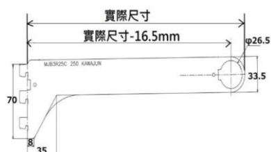
圓管用架手(中央用)
