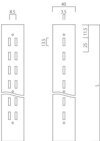
剖面圖
